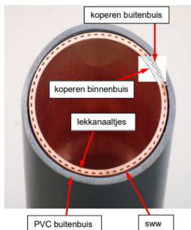
Doorsnede van een concentrische warmtewisselaar
