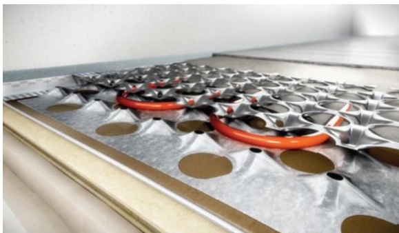
Twee voorgevormde stalen bladen met ertussen verwarmingsbuizen – op de ondergrond gekleefde platen
