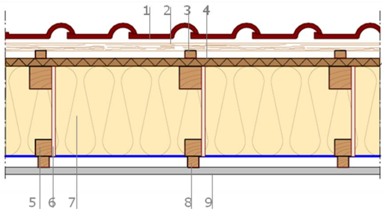
1. dakbedekking – 2. panlatten – 3. tengellatten – 4. winddicht onderdak op bestaande draagstructuur (keperdak) – 5. hulpkepers – 6. dunne plaat – 7. Isolatie – 8. Latwerk – 9. Binnenafwerking (Illustratie: VIBE vzw)
