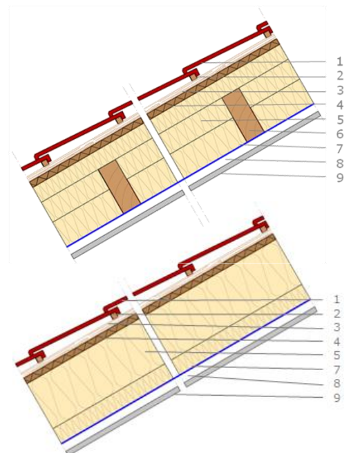
1. Dakbedekking – 2. Panlatten – 3. Tengellatten – 4. winddicht onderdak – 5. isolatie tussen de draagstructuur – 6. Gordingen – 7. Luchtscherm – 8. Leidingsponw – 9. binnenafwerking
