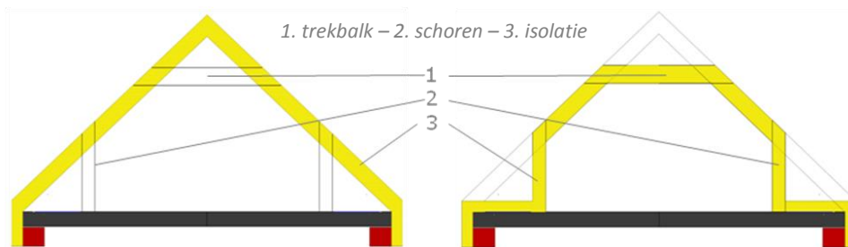
Links: spantendak met isolatie tot in de nok. Rechts: spantendak met isolatie ter hoogte van de trekbalen en de schoren.
