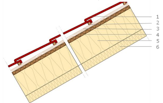
1. dakbedekking – 2. Panlatten – 3. Tengellatten – 4. Winddicht onderdak – 5. 1 e laag isolatie tussen de spanten – 6. 2 e laag isolatie onder de spanten
