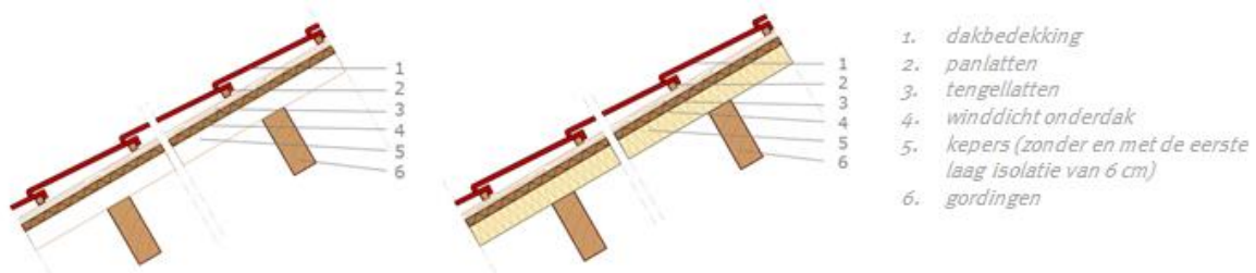
Isoleren van keperdak met eerste laag vlasisolatie tussen de kepers (Foto: E. Willaert)
