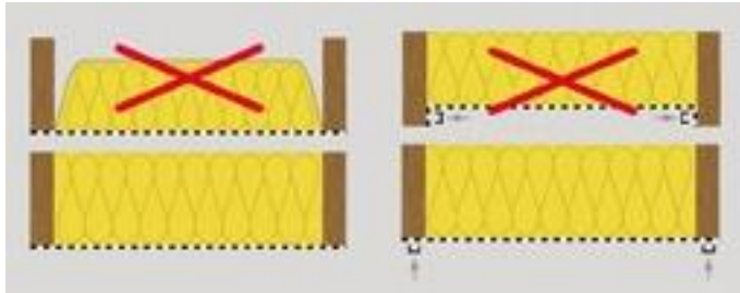
Flensdeks: verkeerde plaatsing (boven) en correcte plaatsing (onder). (illustraties: Isover)
